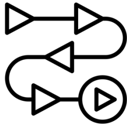
Video Codec
